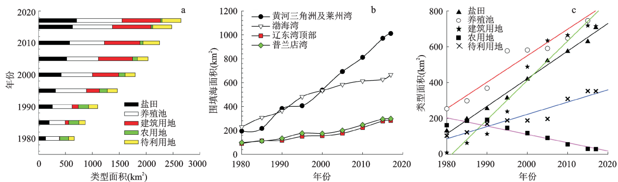
图5 1980~2017年环渤海区域围填海各利用类型面积变化(a)、重点变化区域面积变化(b)及各类型面积演变趋势(c)
